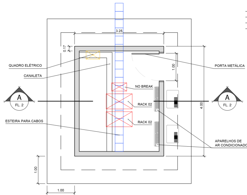
PLANTA ESCALA 1:50
